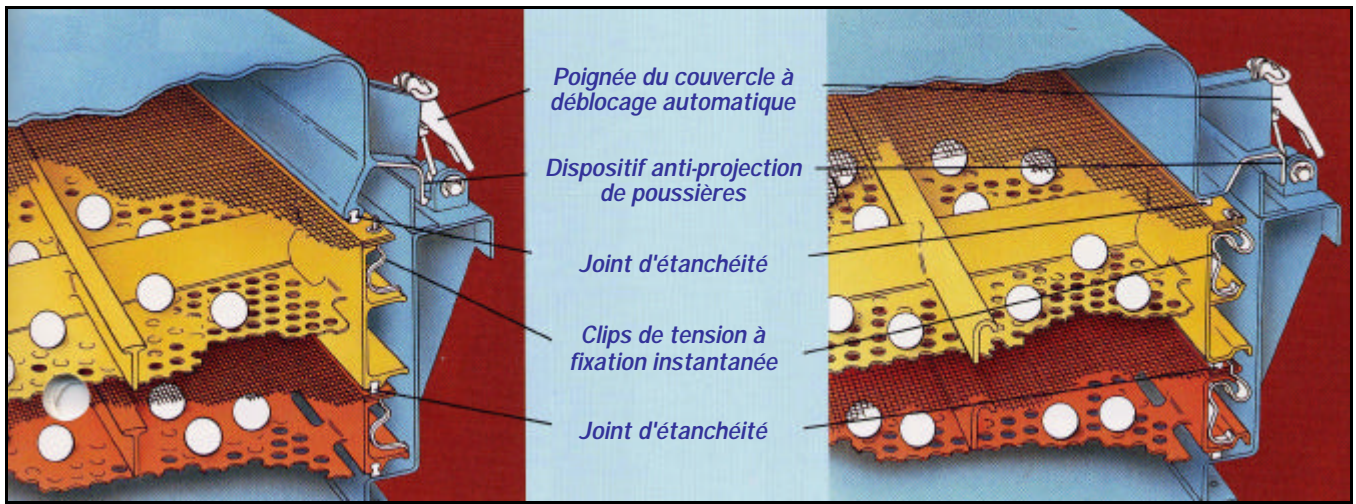
Couvercle et tamis en aluminium
